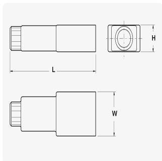
CAPSULE PER TERMINALI FEMMINA DIRITTI 4,8 AD INNESTO POSTERIORE
