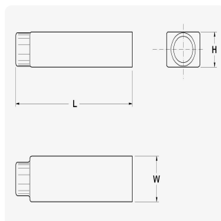
CAPSULE PER TERMINALI FEMMINA DIRITTI 2,8 AD INNESTO POSTERIORE
